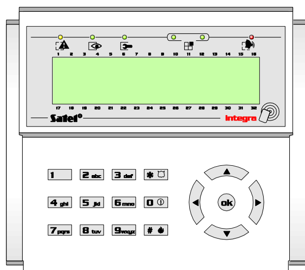
Fig. 1. Betjeningspanel INT-KLCDR-GR.
