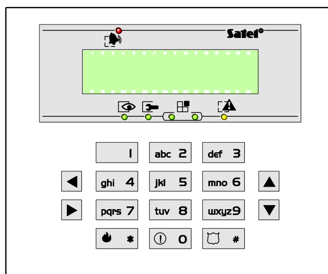
Fig. 2. Betjeningspanel INT-KLCDS-GR.
