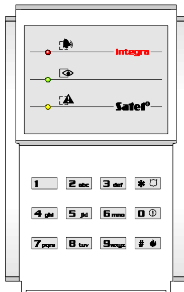
Tegning 4. Områdebetjeningspanel INT-S-GR / INT-S-BL.
